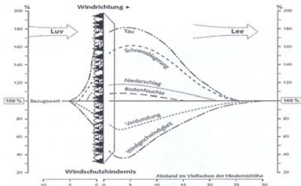
3.3.1 - Abbildung 1 : Reichweite und Wirkungen von Windhindernissen 1
